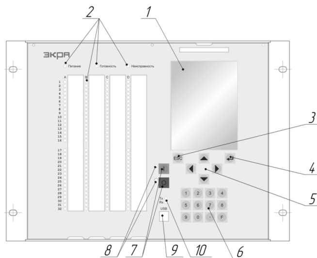
б) терминал типа ЭКРА 2X2(A)
