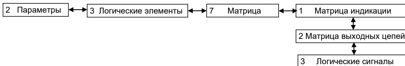
Рисунок 26 – Структура меню Матрица
