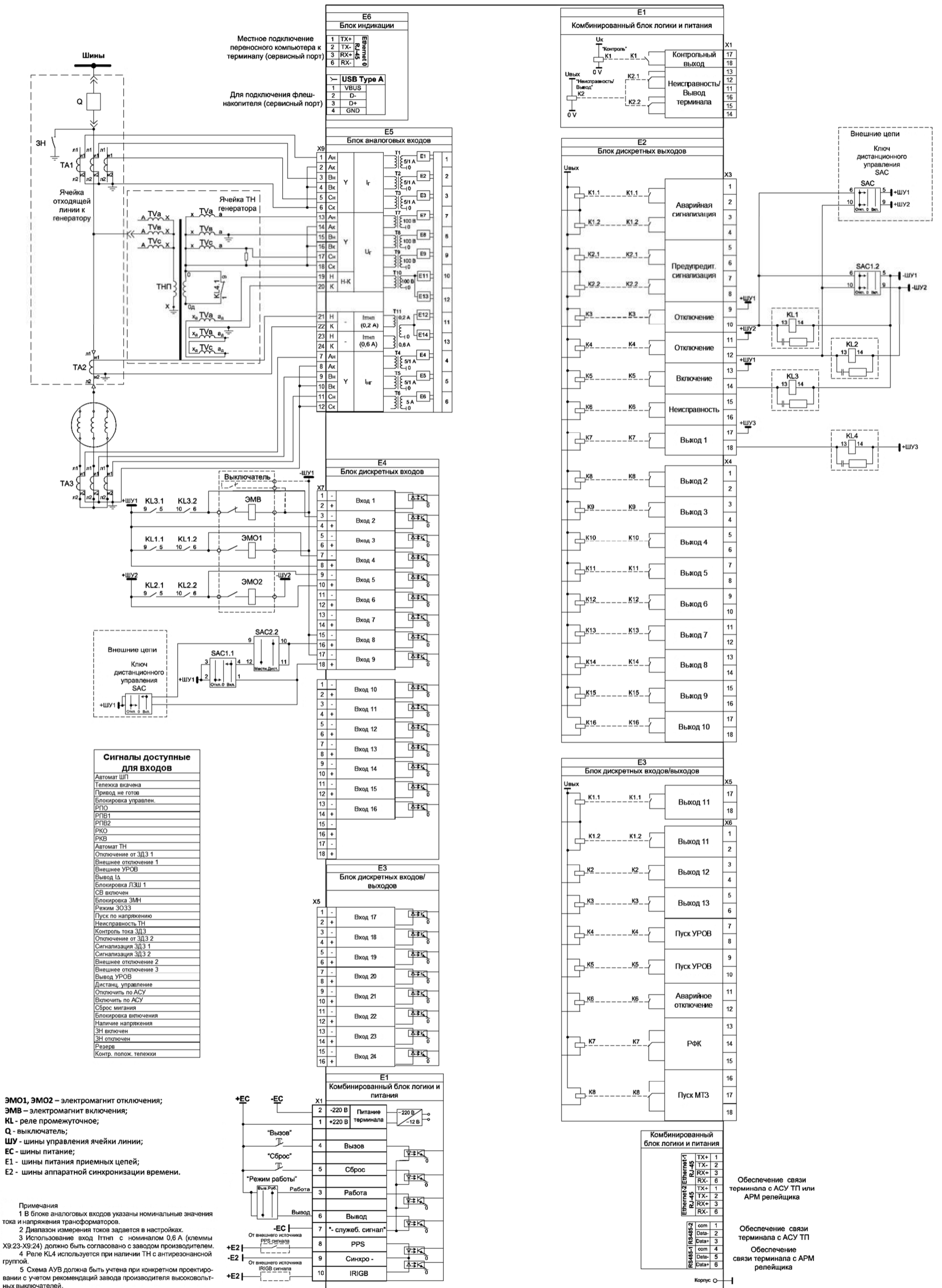
Рисунок Л.1 – Пример подключения внешних цепей к терминалу защиты генератора
