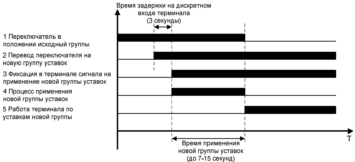
Рисунок 2 – Переключение группы уставок в соседнее положение
