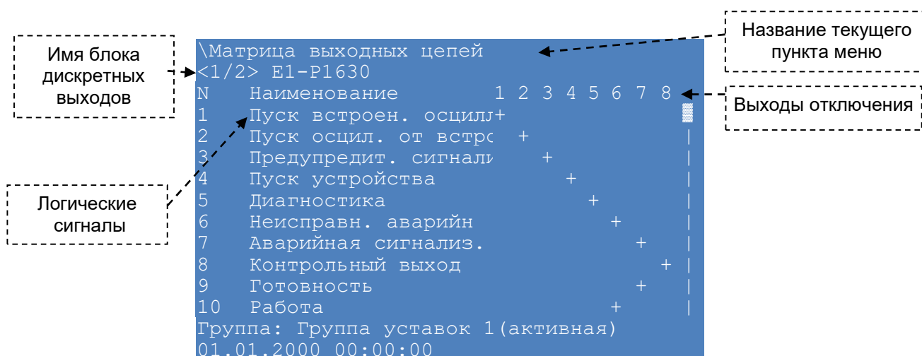
Рисунок 28 – Внешний вид меню Матрица выходных цепей
