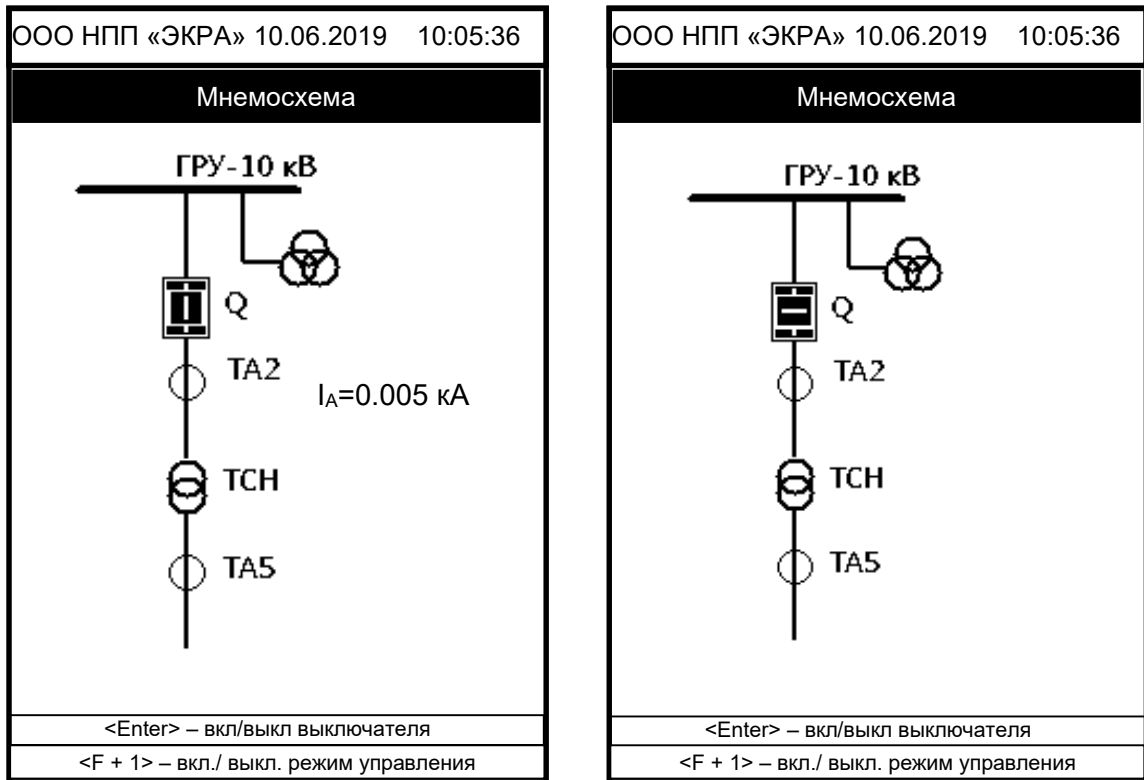
а) включенное положение выключателя
